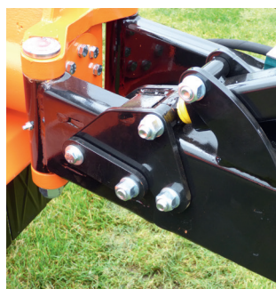
Dispositif anti collision dans les bras de dépo
